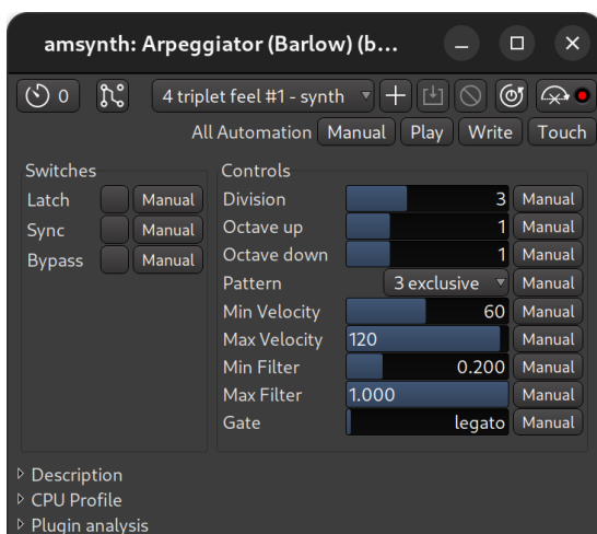
Fig. 76.8 - Barlow arpeggiator
