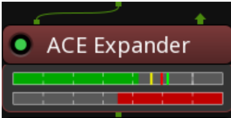
Fig. 74.4 - Inline display
