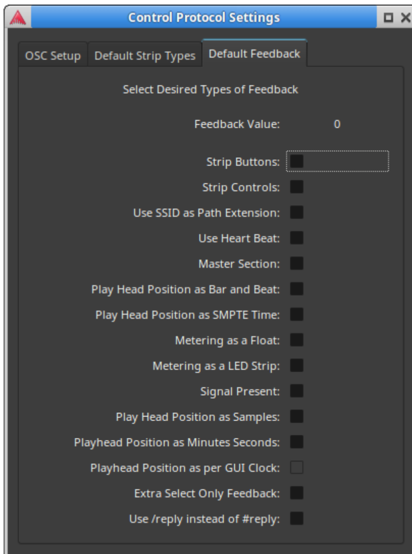
Fig. 82.7 - The Default Feedback tab
